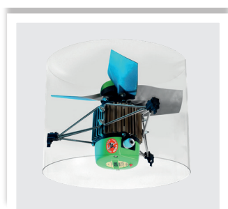
Ventilateur EMI intégrable en cheminée
