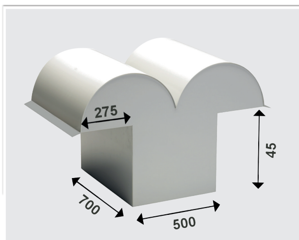
Capot Y en polyéthylène noir ou gris clair
