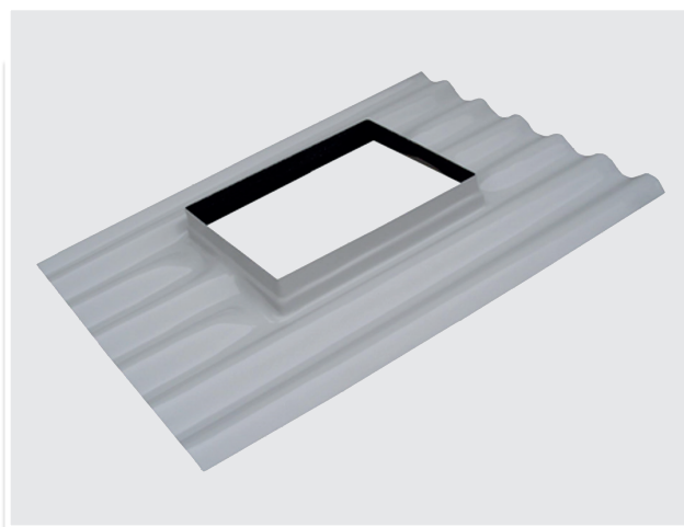
Plaque châssis en polyester 6 ondes 1/2 de 177mm - 1,58m Ouverture 680 x 480 mm
