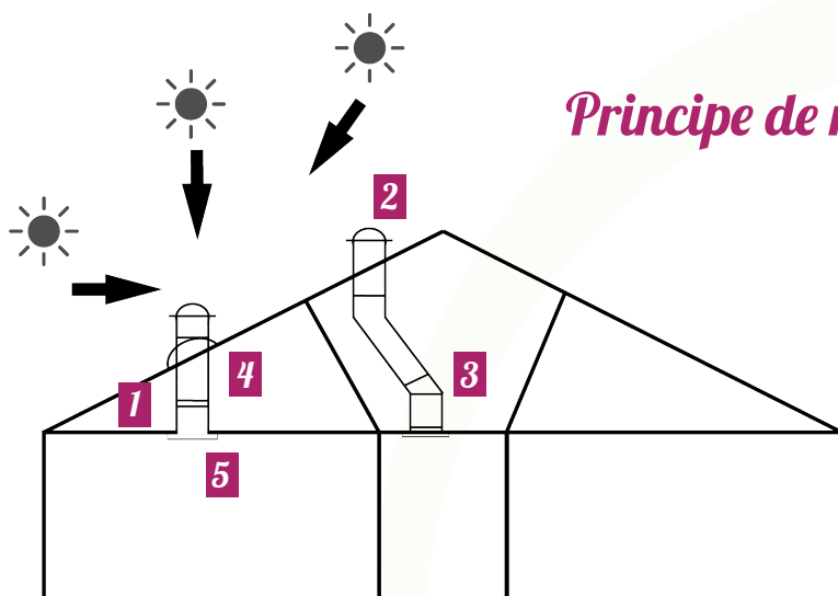
Shéma en coupe type porcherie
